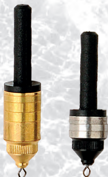
16 g-os súly rézből (bal) és az új ötvözetből (jobb)
